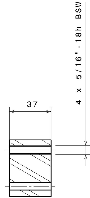
CORTE AA
